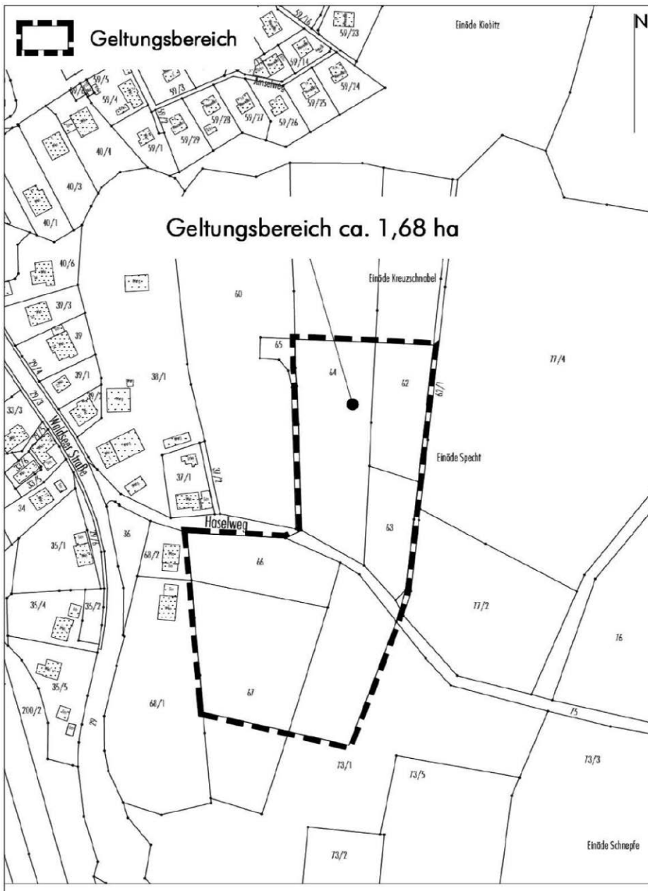
Lageplan maßstabslos
