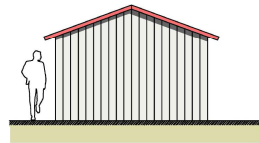
Ansicht Süd
