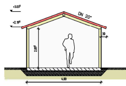
Schnitt
