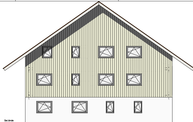
Ansicht West
