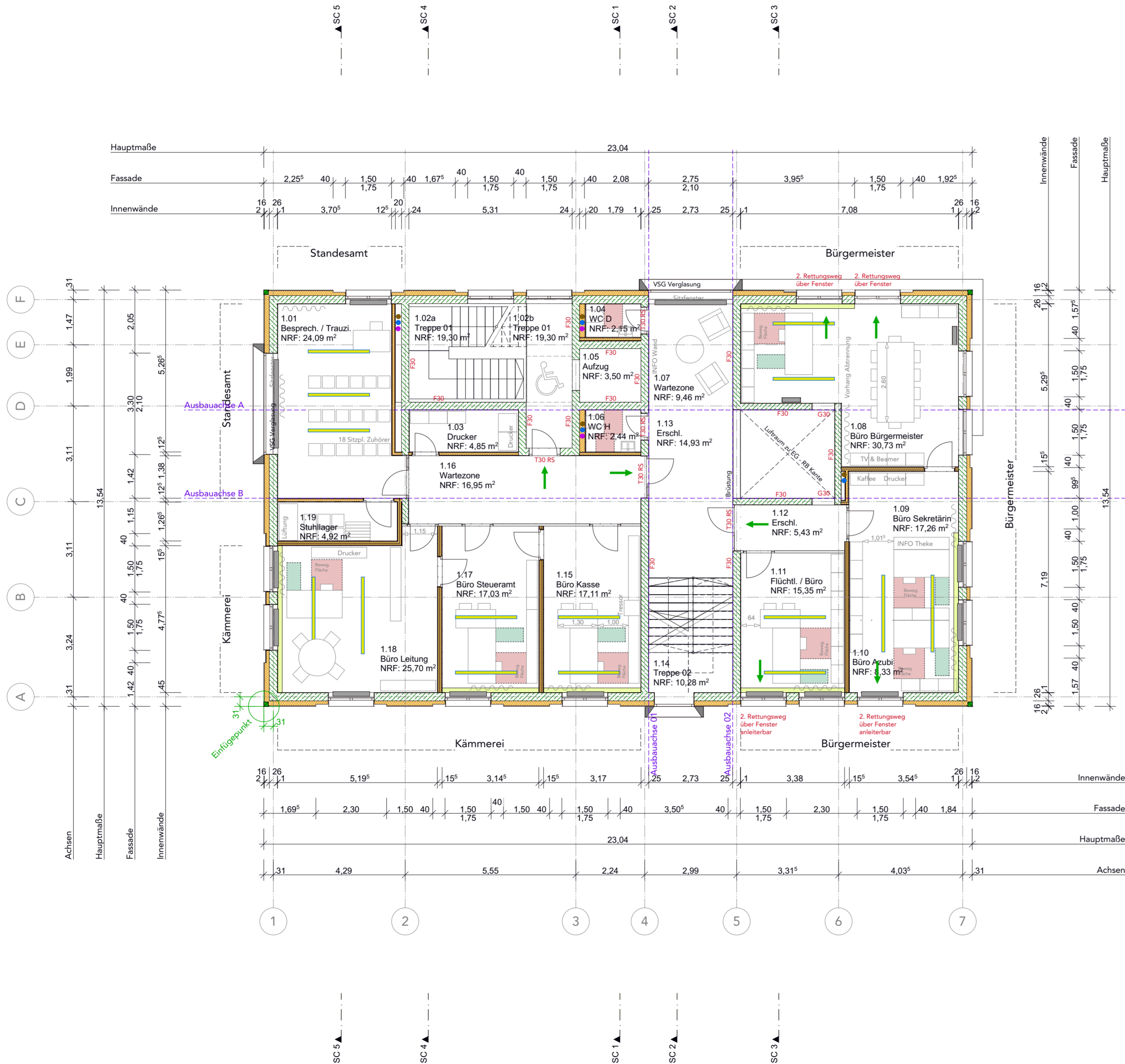
Grundriss OG
